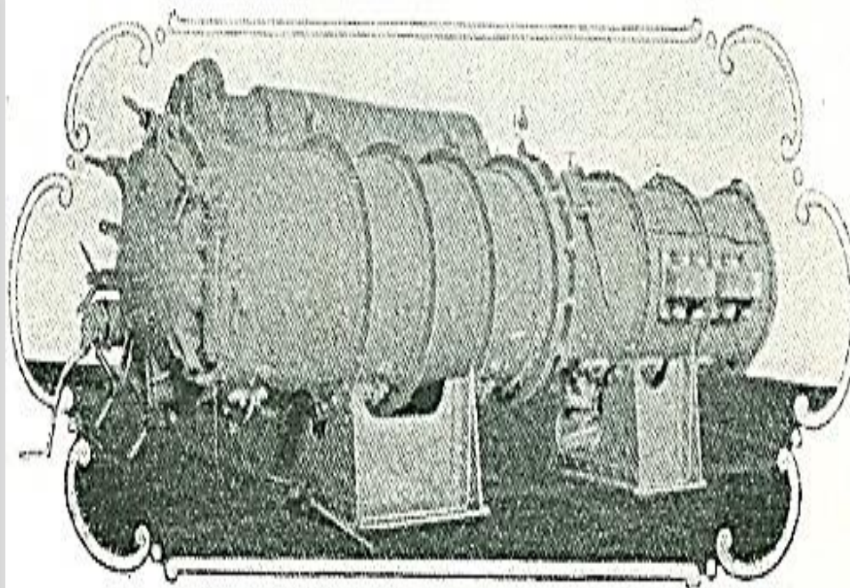
Японская минная пушка для стрельбы минами Уайтхеда.
