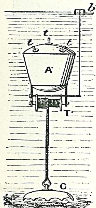
Наша автоматическая мина.
